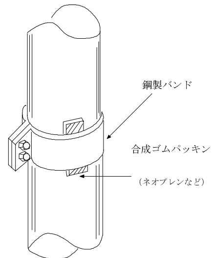
改修例
