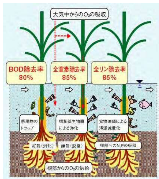
植生浄化法の仕組み
