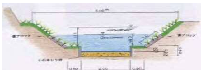
複断面水路
