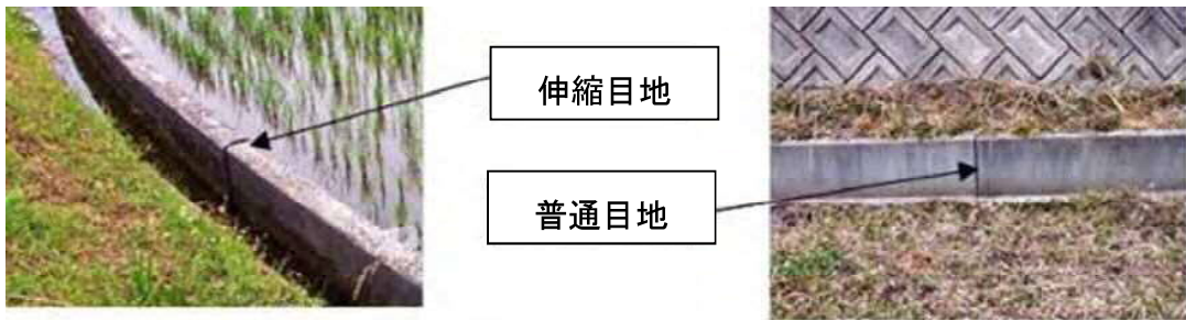
目地の種類
