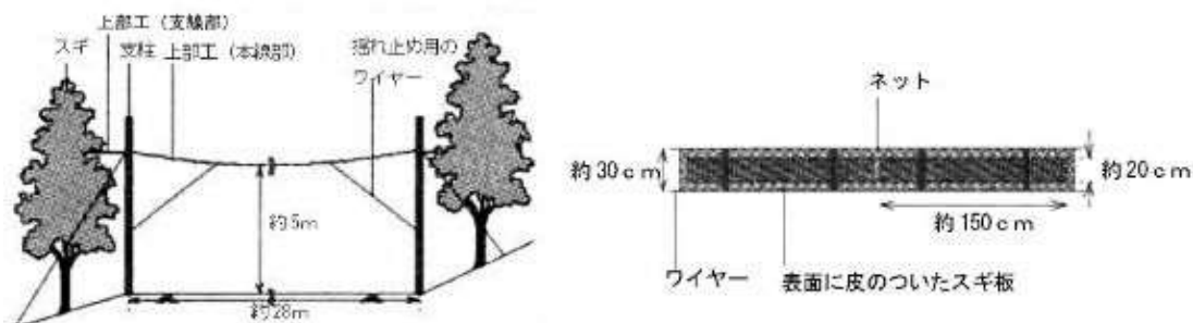
橋梁の構造例（出典：清水建設）
