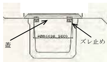
蓋設置例（断面図）
