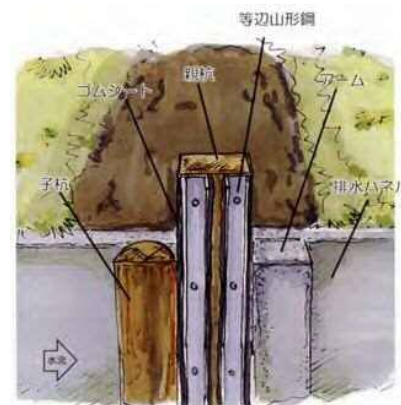
親杭、子杭、レールの設置イメージ （出典：滋賀県 魚のゆりかご 水田プロジェクト）
